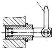
吊环销 GN 1130
